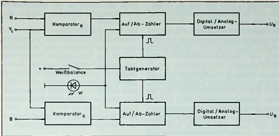
Bild 3. Funktionsprinzip der elektronischen Verstärkungsregelung in den beiden Chrominanzkanälen R und B durch Vergleich mit dem jeweiligen Helligkeitssignal Y_L bei der automatischen Weißbalance-Einstellung
