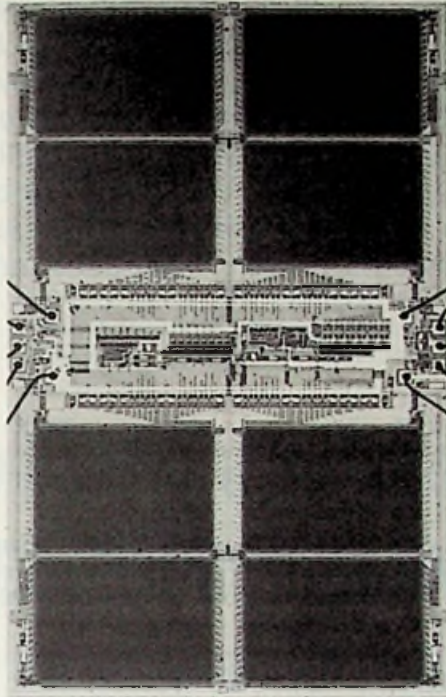
Bild 6: Chipfoto des 300 Kbit CCD-Speichers für Bildspeicheranwendungen
