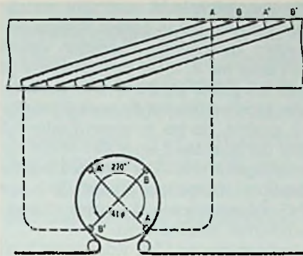
Bild 3. Kopfradumschlingung und Spurverlauf auf dem Magnetband bei VHS-Video movie
