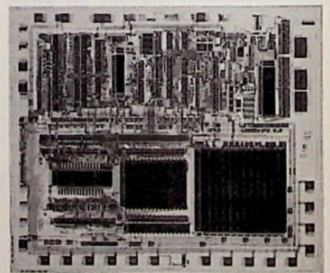
Bild 5: Chipfoto des Btx-IC's EUROM, Typ SAA 5350
