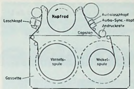
Bild 4. a) ▲ Bandverlauf im klassischen VHS-Video recorder. Der Kopftrommeldurchmesser ist nicht maßstabsgetreu b) Bandverlauf im VHS-Video movie ▼
