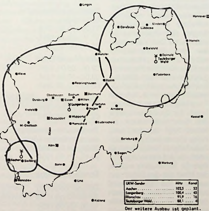
Bild 1: Empfangsbereiche der UKW-Sender mit dem 4. Programm
