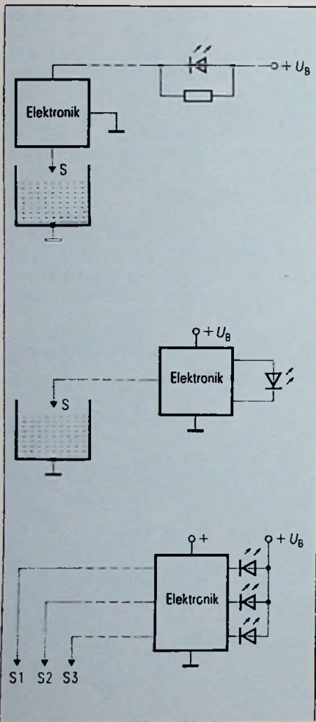
Bild 3: Systemvarianten des Wassersensors; a) Elektronik und Sensor sind zu einer Baugruppe zusammengefaßt, die Anzeige-LED ist räumlich abgesetzt; b) Elektronik und Anzeige-LED sind eine Baugruppe, der Sensor ist abgesetzt; c) Elektronik und Anzeige-LED als Zentralelektronik für mehrere, abgesetzt betriebene Sensoren (S1, S2, S3)
