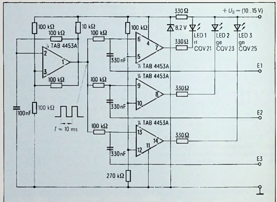
Bild 4: Dimensionierte Schaltung für die Möglichkeit nach Bild 3c
