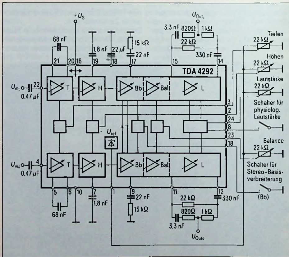
Bild 2: Blockschaftbild des TDA 4292 mit Außenbeschaltung
