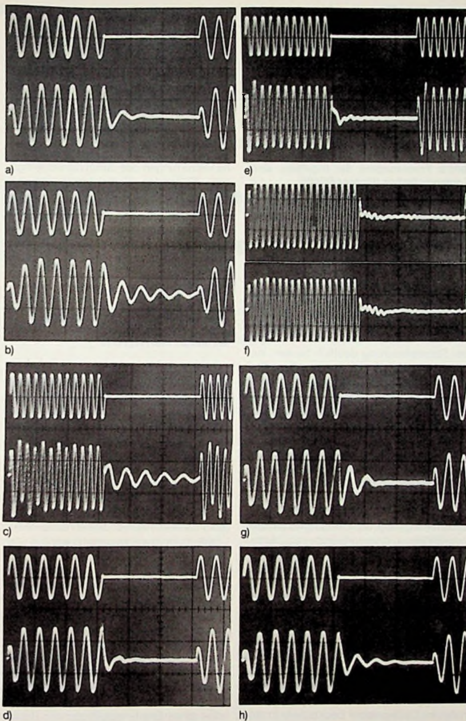
Bild 6: Schirmbildaufnahmen des Einschwingverhaltens bei Steuerung mit einer getasteten Sinusschwingung
