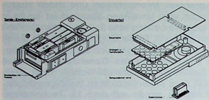
Bild 1: Aufbau des Teleport 9 ▲
