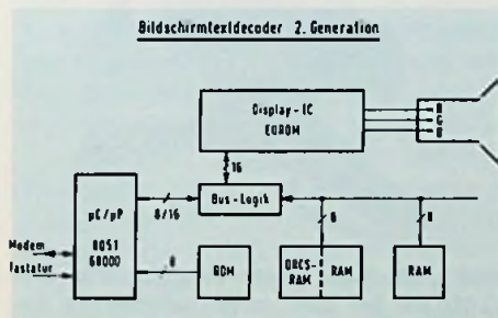
Bild 1: Bildschirmtextdecoder der 2. Generation
