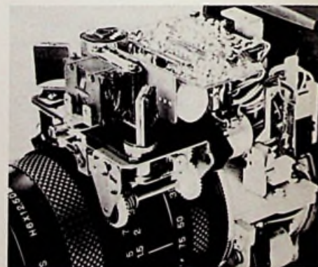
Bild 2. Die Anordnung der Auto Focus-Einrichtung oberhalb des Zoom Objektivs. Links oben: feststehender, rechts vorn: oszillierender Schwingenspiegel, mitte: das optische Umlenkensystem zum dahinterliegenden Doppel-Fotosensor, unten: Servoelektronik mit Getriebemotor
