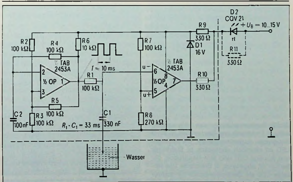
Bild 2: Schaltung des Wassersensors mit Doppel-OP (TAB 2553A)
