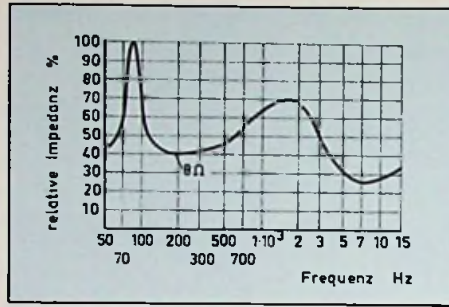
Bild 8: Frequenzgang der Impedanz einer Lautsprecherbox (Pioneer CS565)
