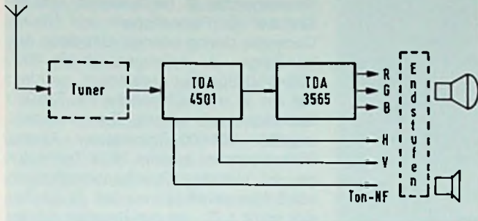
Bild 1: 2 IC-Farbfernseher Konzept, TDA 4501 ZF- und Ton-Signal-Verarbeitung sowie Synchronisation, TDA 3565 PAL-Decoder und Videoprozessor
