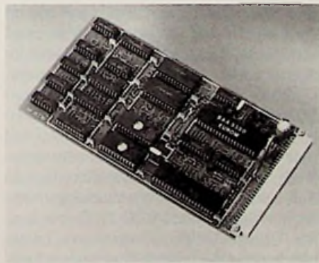
Bild 2: Praktischer Einschub eines Btx-Decoders mit dem neuen EUROM SAA 5350 (Valvo-Pressbild)
