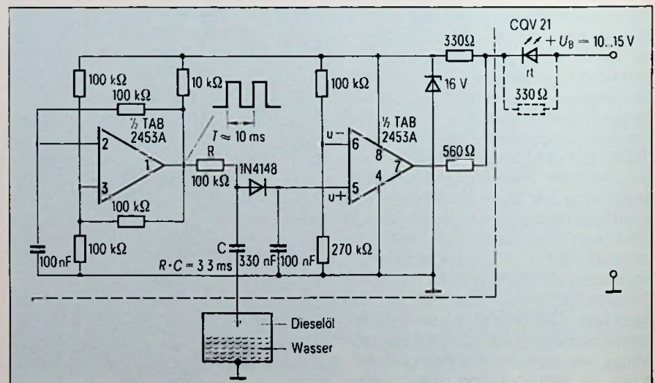
Bild 5: Schaltung eines Wassersensors für Dieselmotoren mit dem Doppel-Operationsverstärker TAB 2453A
