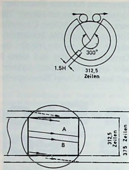
Bild 1. Kopfrad-Umschlingung und Spurverlauf auf dem Magnetband bei Betamovie
