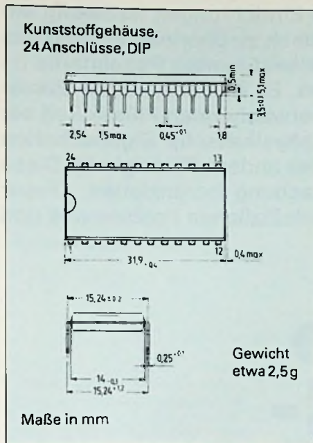
Bild 3: Gehäuseabmessungen des TDA 4292
