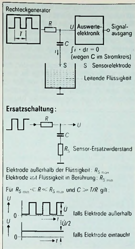
Bild 1: Prinzipanordnung des elektronischen Wassersensors mit Auswerteelektronik sowie Ersatzschaltung
