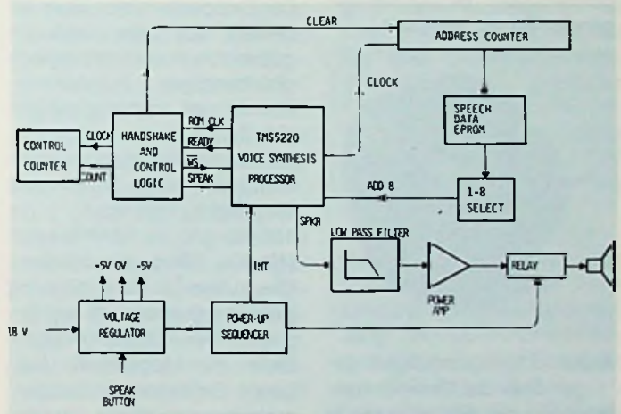
Bild 1: Blockschaltung des Sprachausgabemoduls von TI
