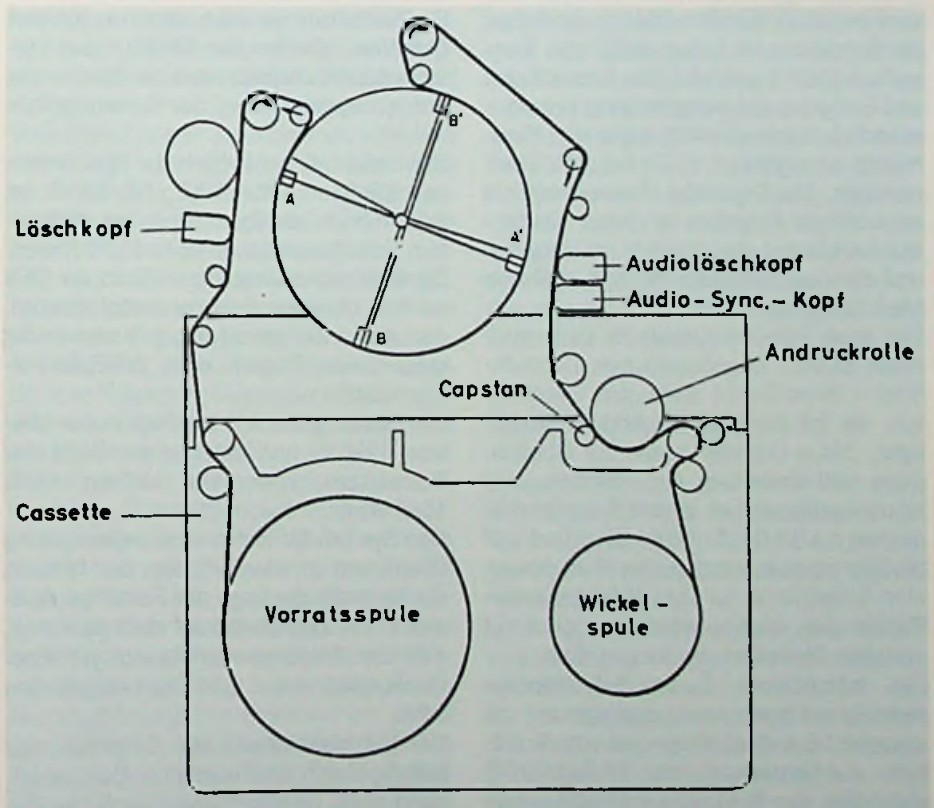
Bild 4. a) ▲ Bandverlauf im klassischen VHS-Video recorder. Der Kopftrommeldurchmesser ist nicht maßstabsgetreu b) Bandverlauf im VHS-Video movie ▼
