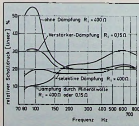
Bild 7: Schalldruck in Abhängigkeit von der Frequenz bei verschiedenen Betriebsarten
