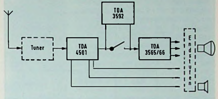
Bild 2: 3 IC-Multistandard-Fernseher, TDA 3592 SECAM-PAL-Transcoder
