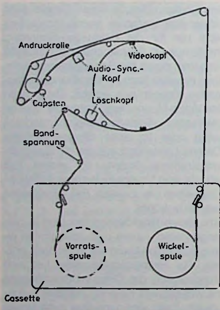
Bild 2. a) Bandverlauf im klassischen Beta-Videorecorder ▲
