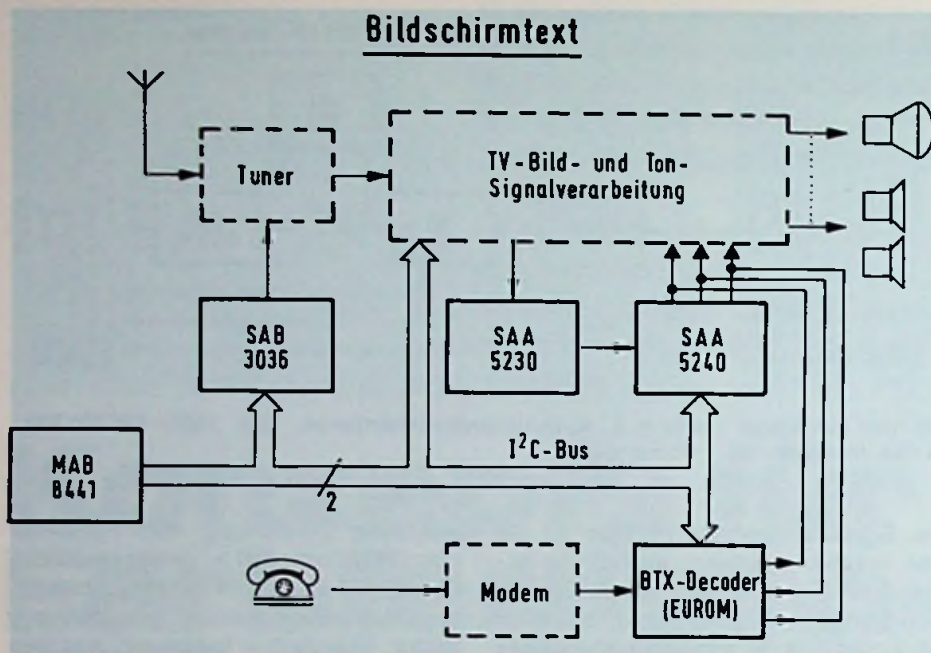
Bild 4: Farbfernsehsystem mit Videotext und Bildschirmtext
