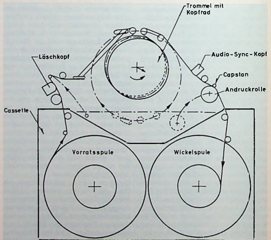
Bild 2. a) Bandverlauf im klassischen Beta-Videorecorder ▲
